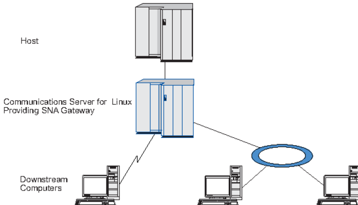
Abbildung 7. SNA Gateway
