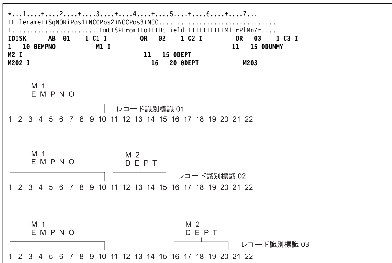
図 3-50. ダミー M2 フィールドによる突き合わせフィールド
