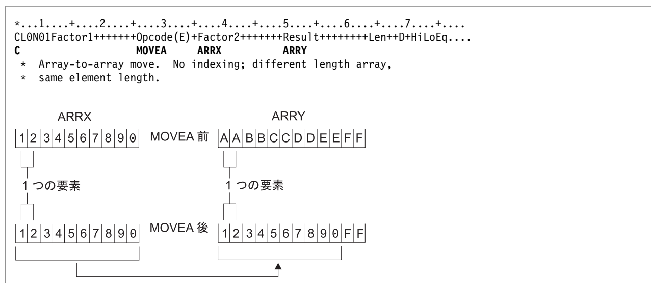
図 6-177. MOVEA 命令
