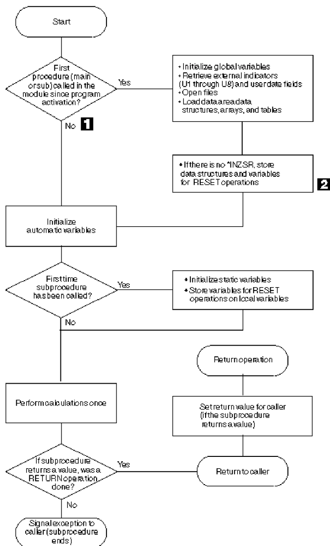
図 3-16. サブプロシーチャーの通常の処理順序
