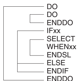
図 6-14. ネストされた構造化グループ
