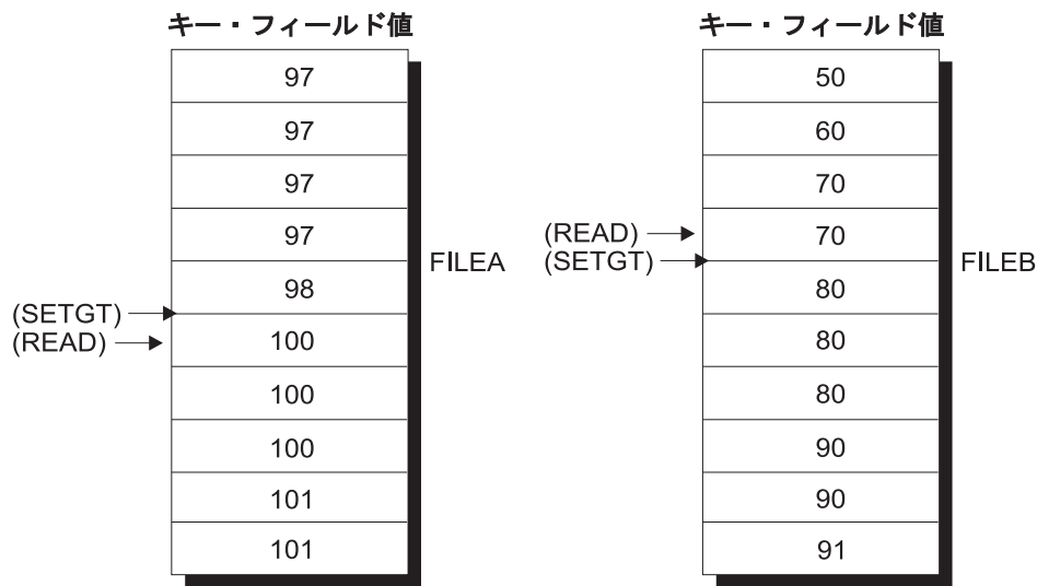
図 6-208. SETGT 命令
