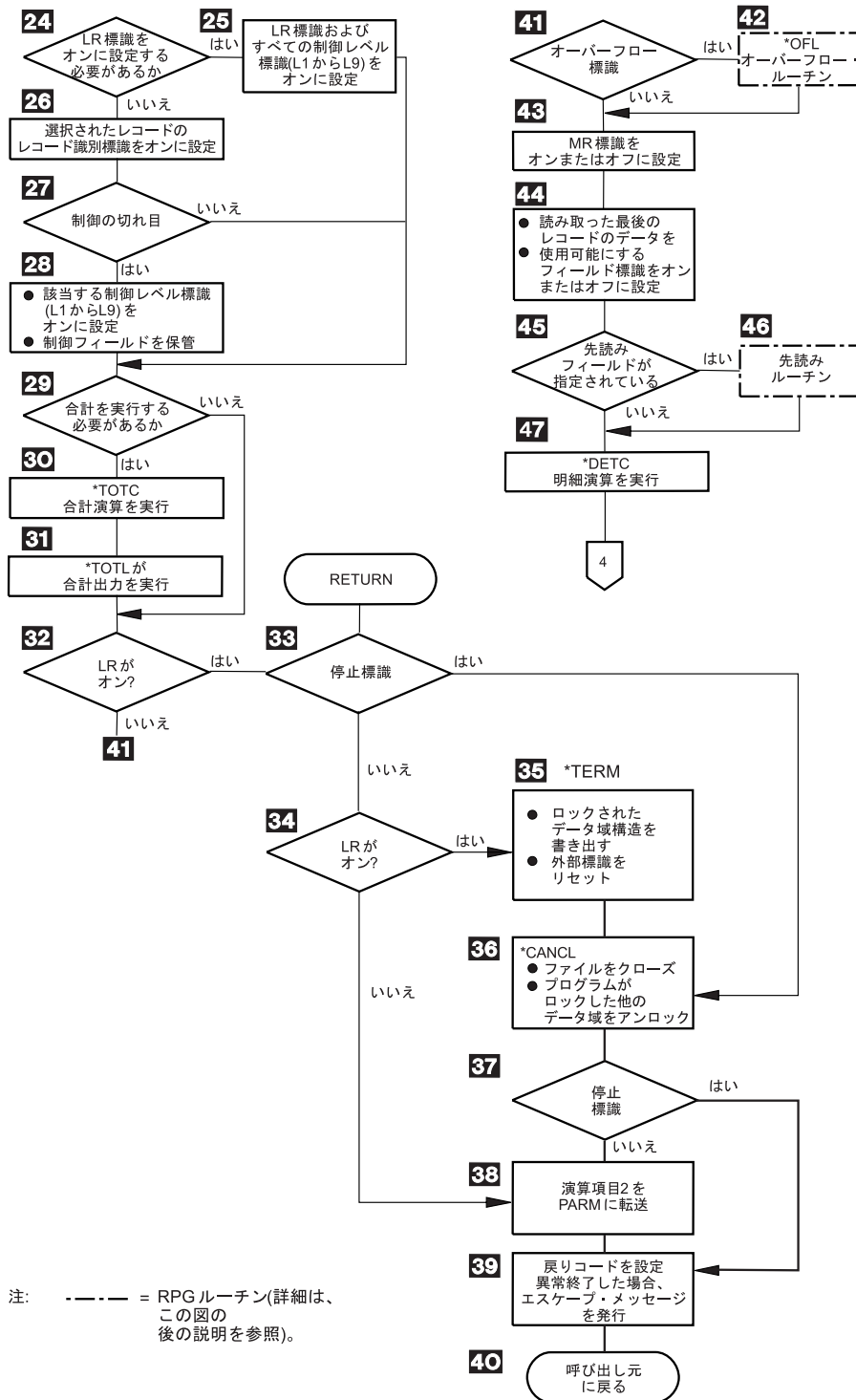
図 8. 詳細な RPG IV オブジェクト・プログラム・サイクル (2/2)
