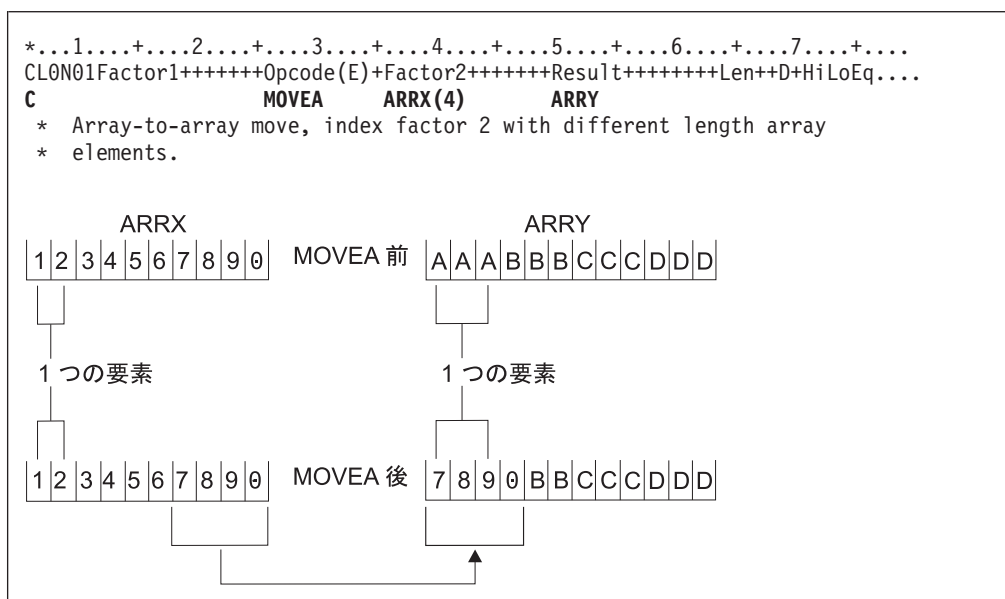
図 346. MOVEA 命令 (4/10)
