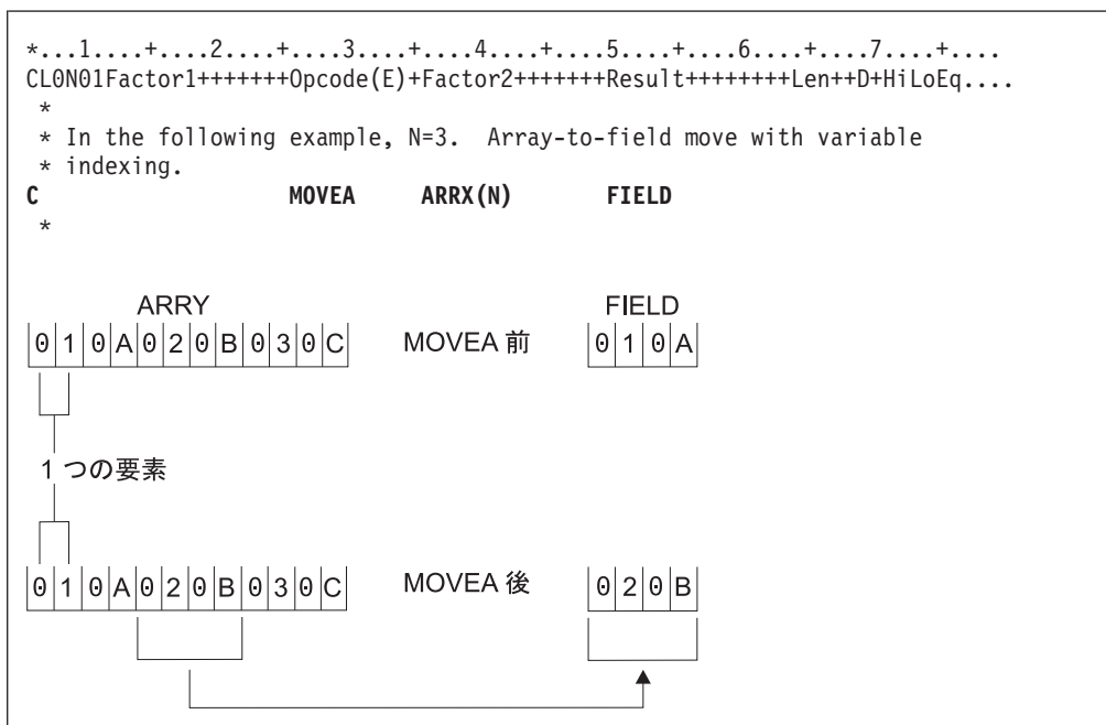
図 346. MOVEA 命令 (6/10)
