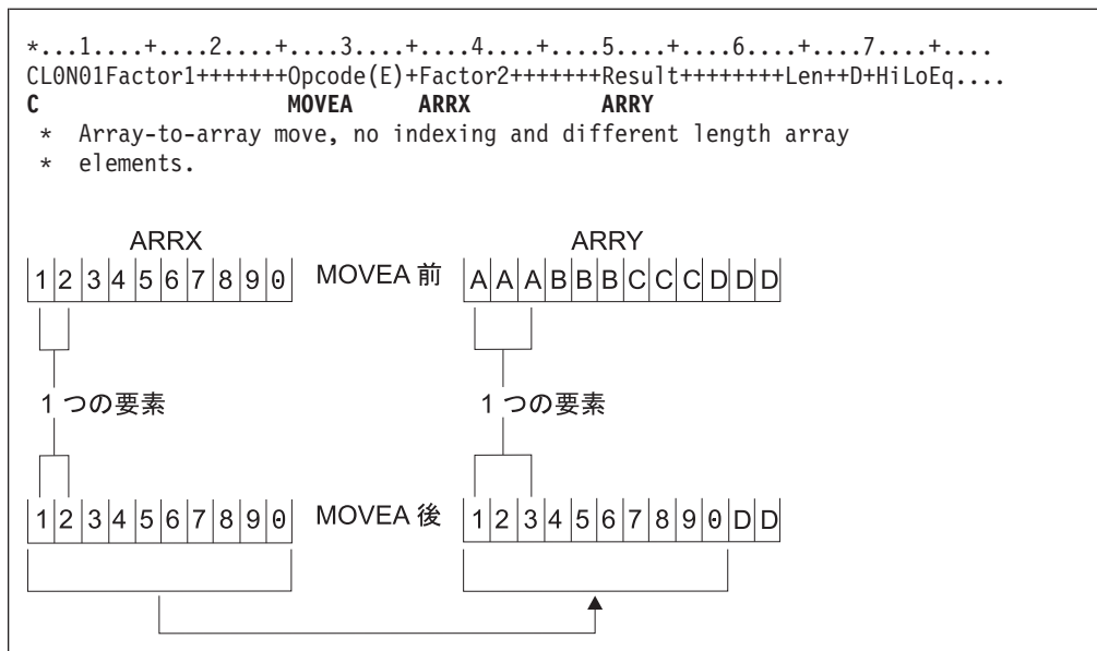
図 346. MOVEA 命令 (3/10)
