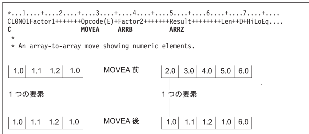
図 346. MOVEA 命令 (7/10)
