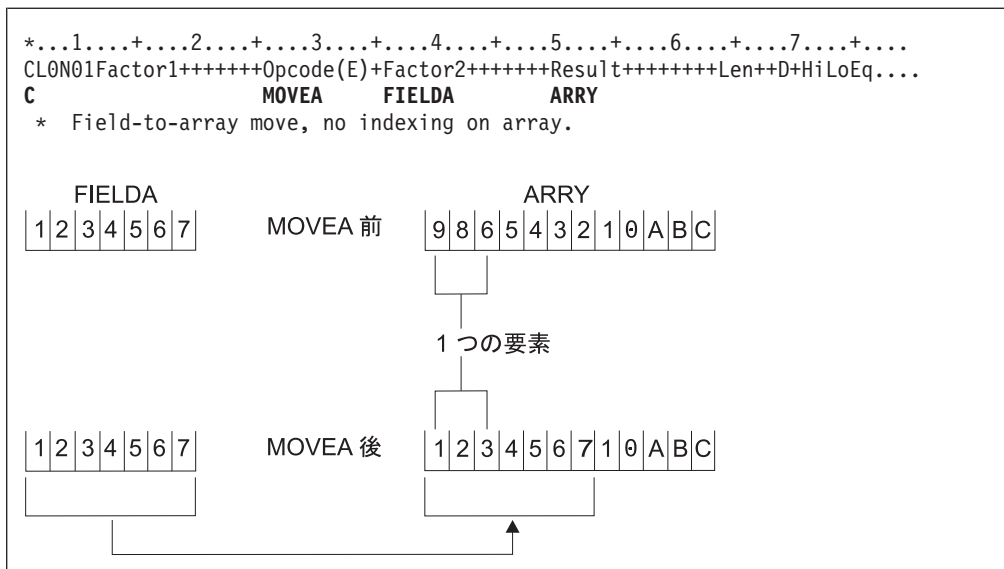
図 346. MOVEA 命令 (5/10)
