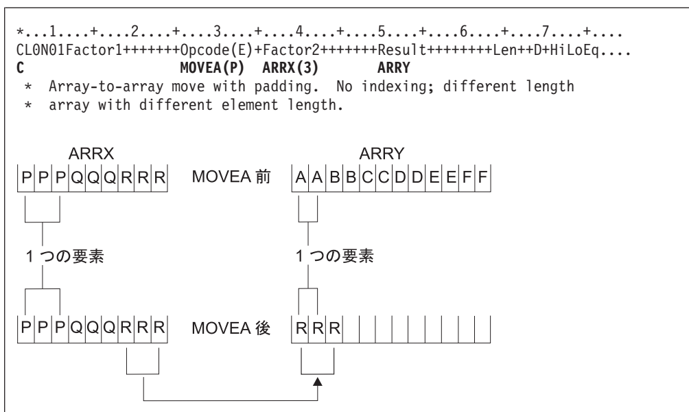
図 346. MOVEA 命令 (10/10)
