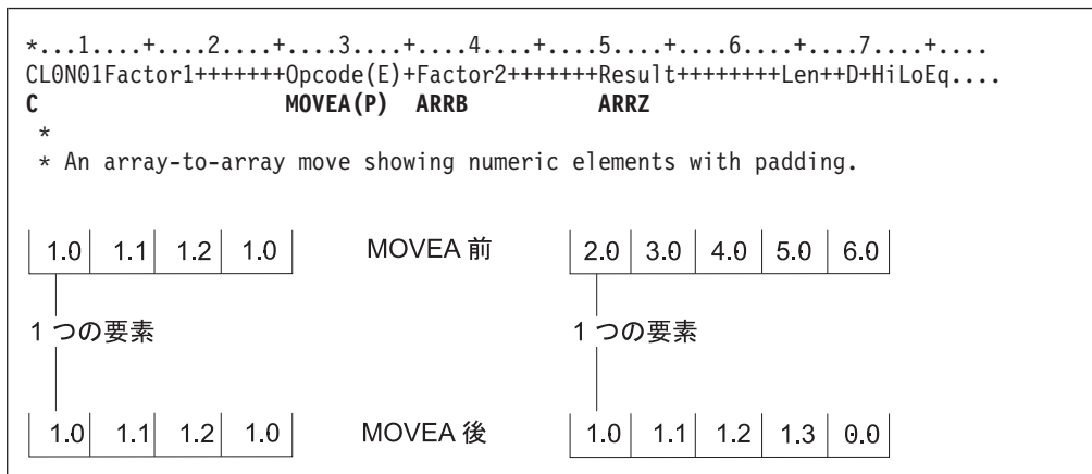
図 346. MOVEA 命令 (9/10)
