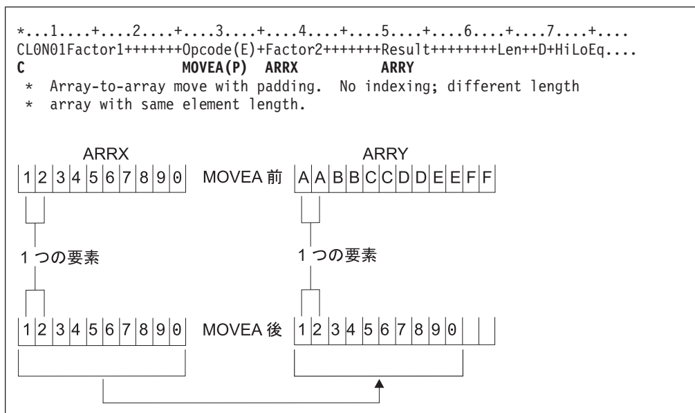
図 346. MOVEA 命令 (8/10)
