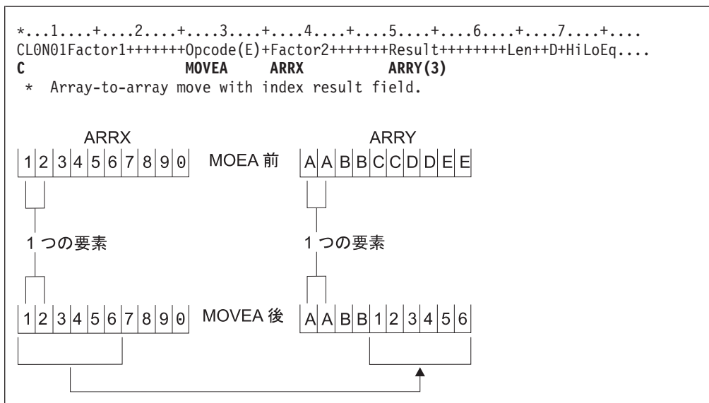
図 346. MOVEA 命令 (2/10)
