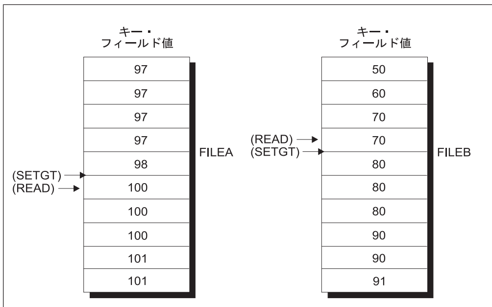
図 377. SETGT 命令 (2/4)
