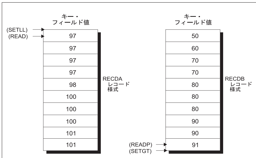
図 377. SETGT 命令 (4/4)
