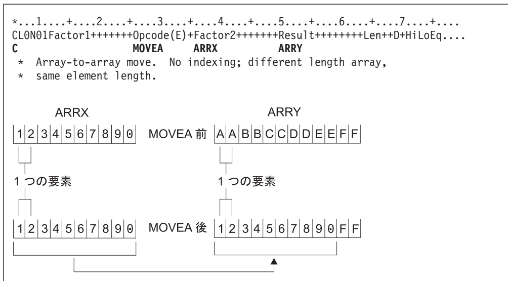
図 346. MOVEA 命令 (1/10)
