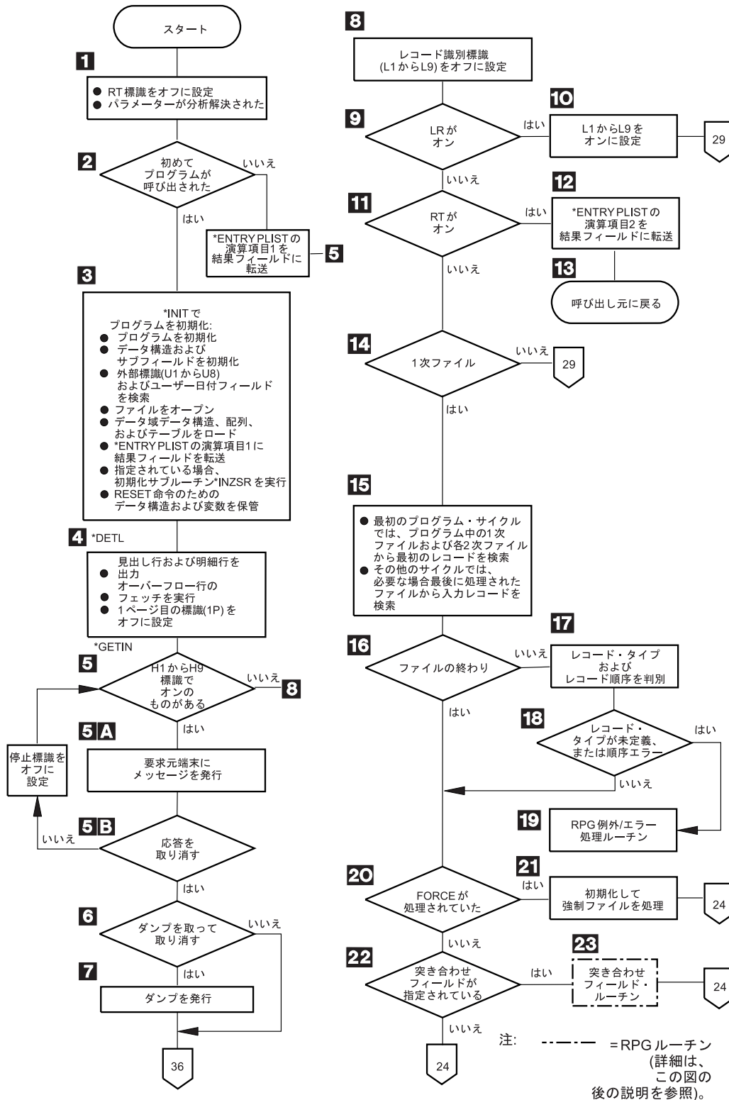
図 8. 詳細な RPG IV オブジェクト・プログラム・サイクル (1/2)
