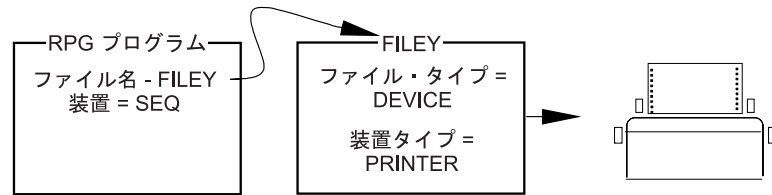
図 155. ファイル名と表示装置ファイル記述との関連付け
