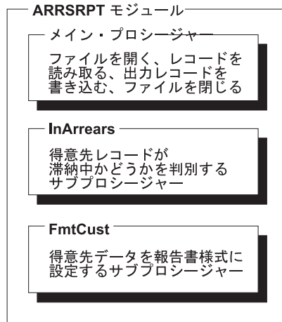
図 17. ARRSRPT モジュールの構成要素
