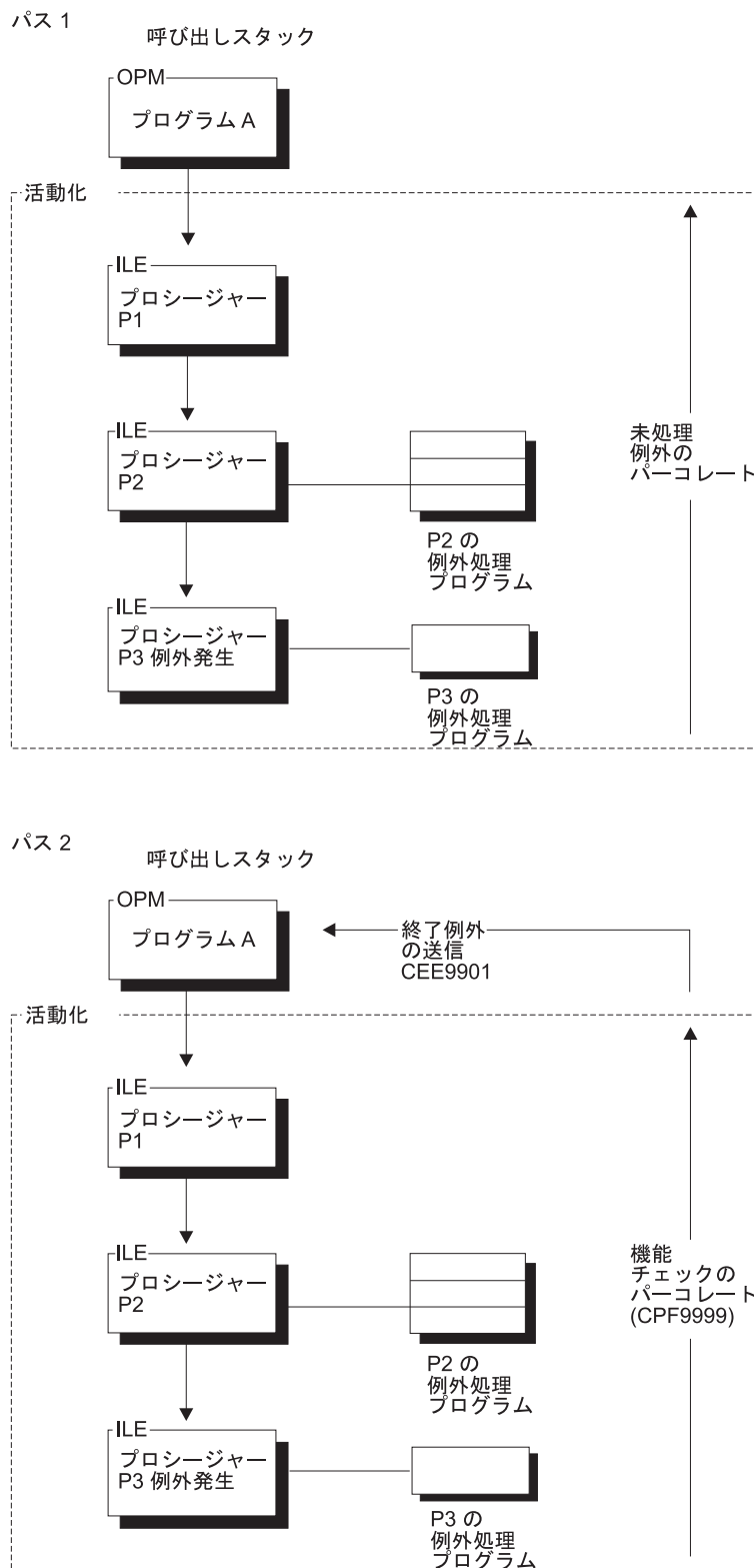
図 134. 呼び出しスタックおよび例外メッセージのパークレーション
