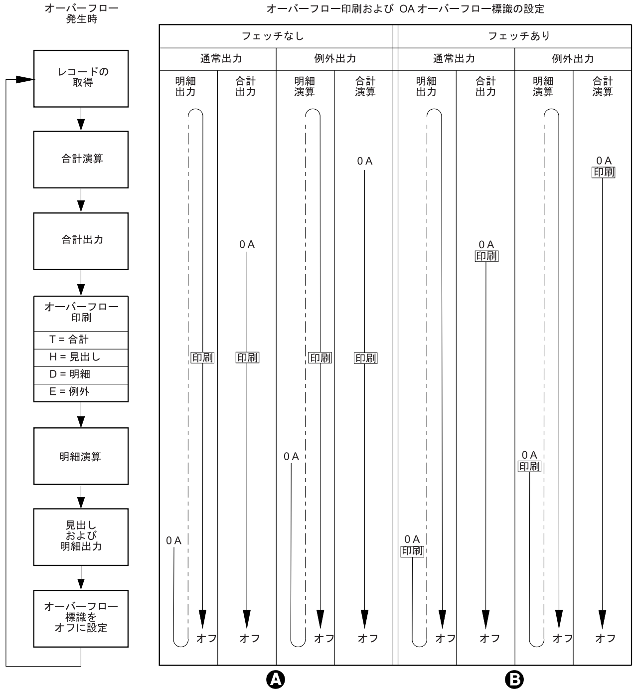
図 186. オーバーフロー印刷: オーバーフロー標識の設定
