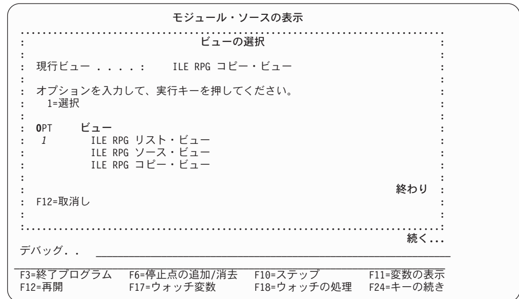
図 106. モジュールのビューの変更
