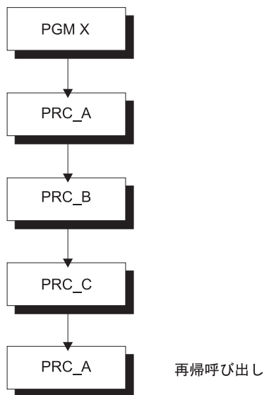
図 62. 避けるべき再帰呼び出しスタック
