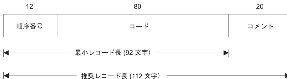
図 220. RPG IV レコード長の説明
