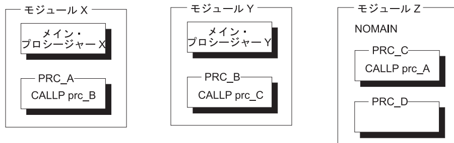
図 61. それぞれがサブプロシージャをもつ 3 つのモジュール
