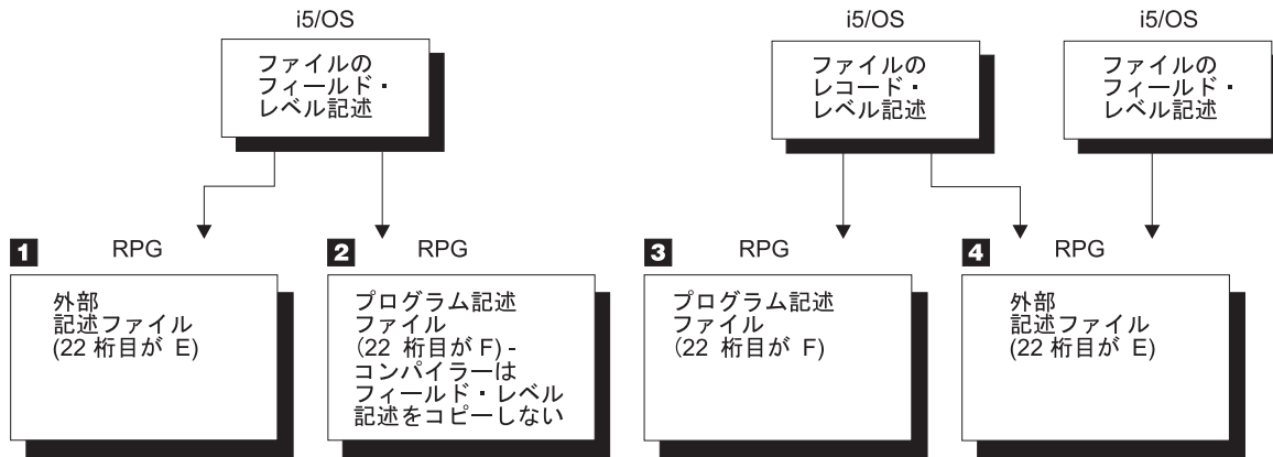
図 156. i5/OS システムでの RPG プログラムとファイル間の代表的な関係
