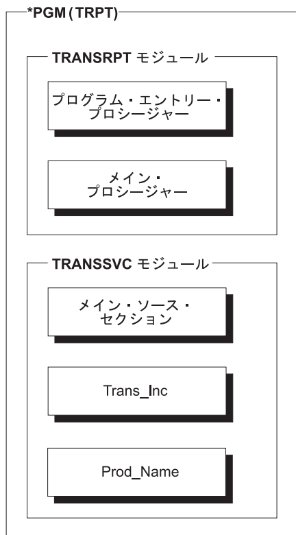
図 41. プログラム TRPT の構造
