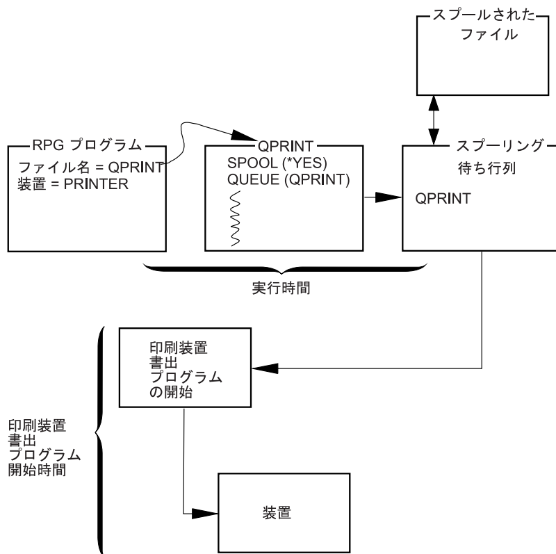
図 165. 出力スプーリング例
