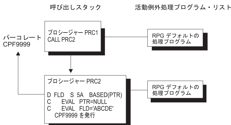
図 136. 処理不能の機能チェックのシナリオ
