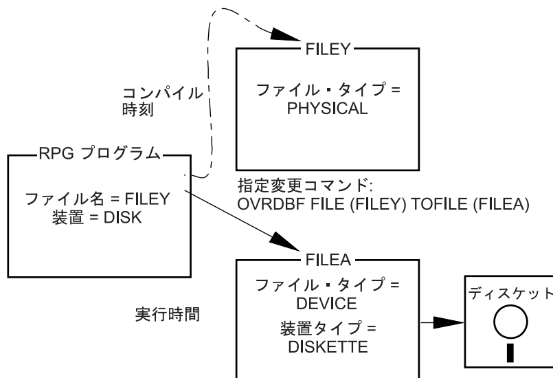
図 163. ファイル入出力の一時変更例
