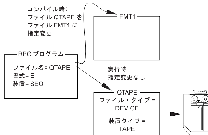
図 164. ファイル入出力の指定変更例
