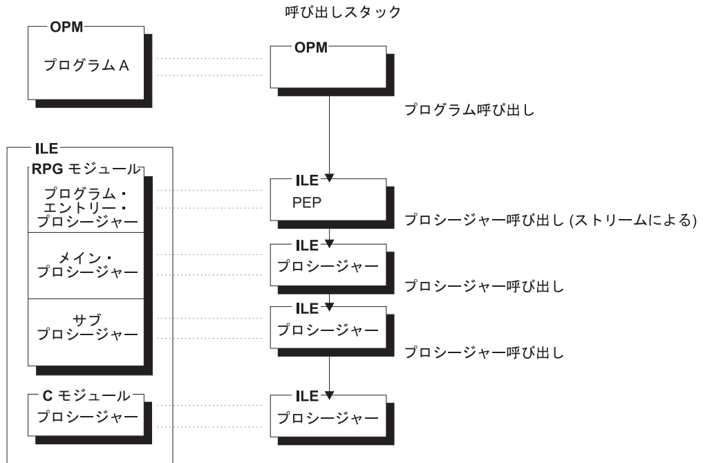
図 60. 呼び出しスタック上のプログラム呼び出しとプロシージャー呼び出し
