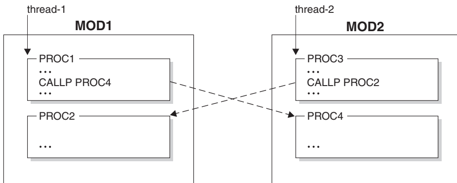
図 75. THREAD(*SERIALIZE) モジュールのデッドロック例
