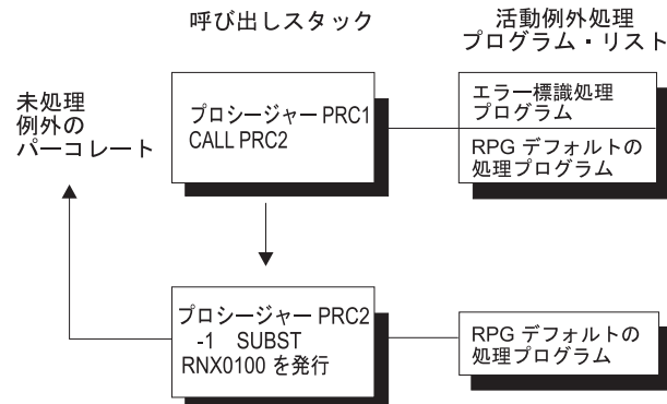
図 135. 処理不能エスケープ・メッセージのシナリオ
