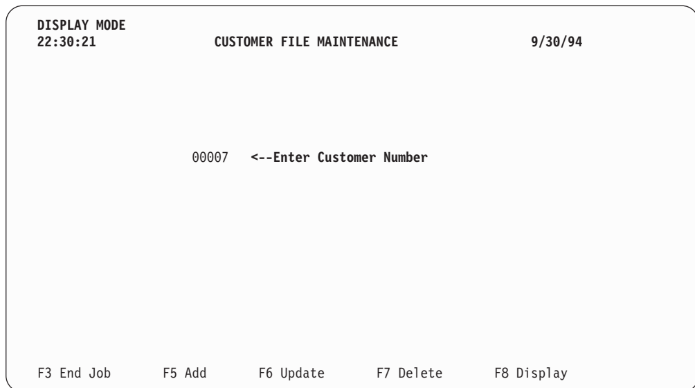
図 203. 'CUSTOMER FILE MAINTENANCE' (得意先ファイル維持) 表示モード・プロンプト画面
