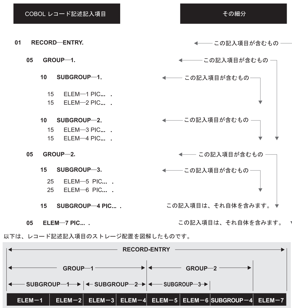
図5. レコード記述のレベル
