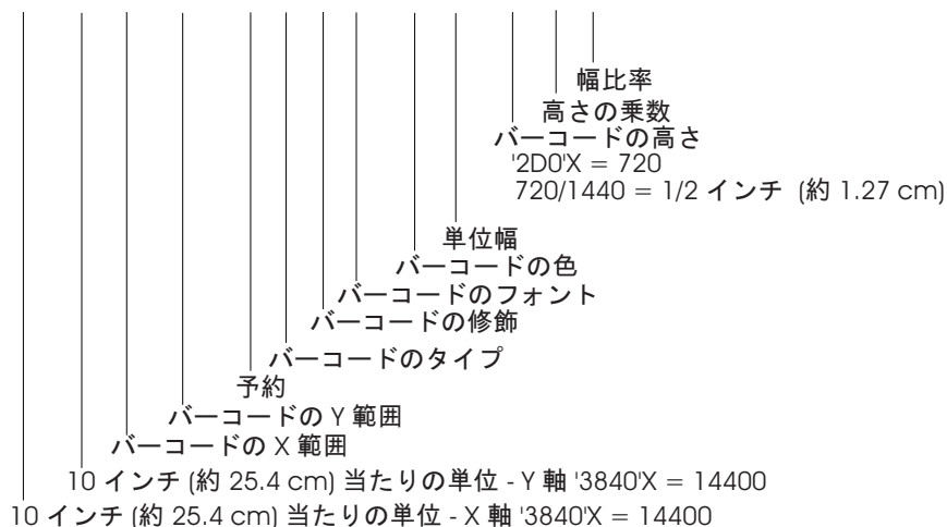
図 4. CVTDTA を使用するバーコード・コマンドのコマンド形式 (1/2)
