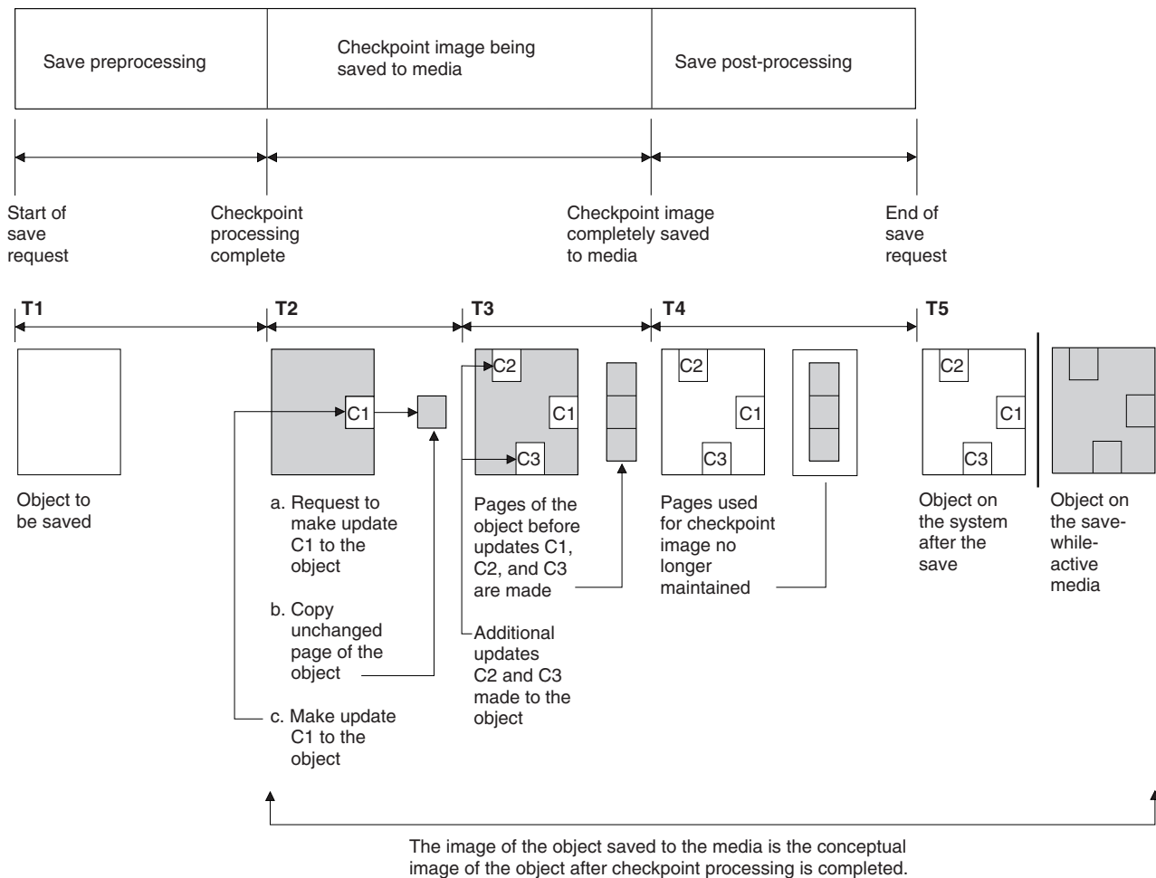
図 6. チェックポイント処理完了後のオブジェクトに対する更新操作のシステム管理
