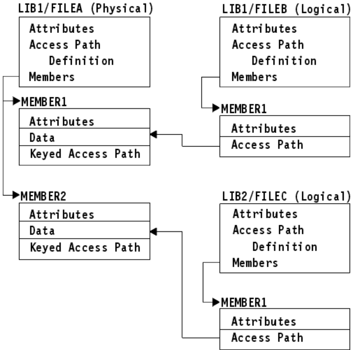
図2. アクセス・パスを保管する
