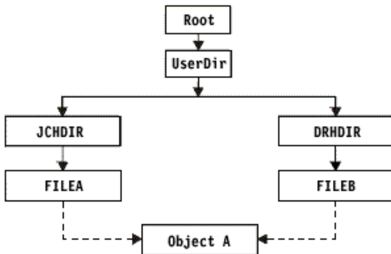
図3. ハード・リンクをもつオブジェクトの例
