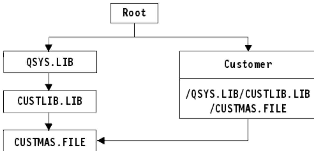
図4. シンボリック・リンクをもつオブジェクトの例
