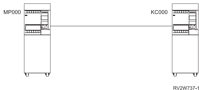
図 20. システムが 2 つの場合のリレーショナル・データベース・ディレクトリーのセットアップ
