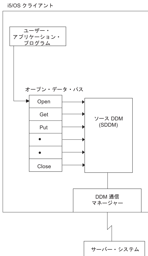
図 13. DDM クライアント・システムとしての i5/OS
