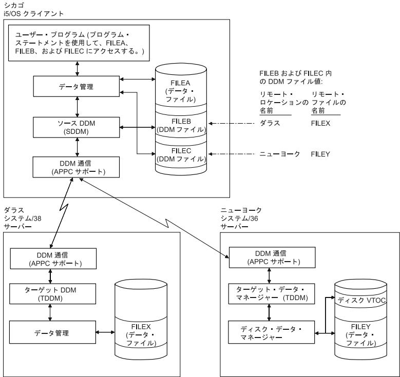
図 18. 例: 複数のローカルおよびリモート・ファイルへのアクセス: システム/38 およびシステム/36 との通信リンクを持った i5/OS。
