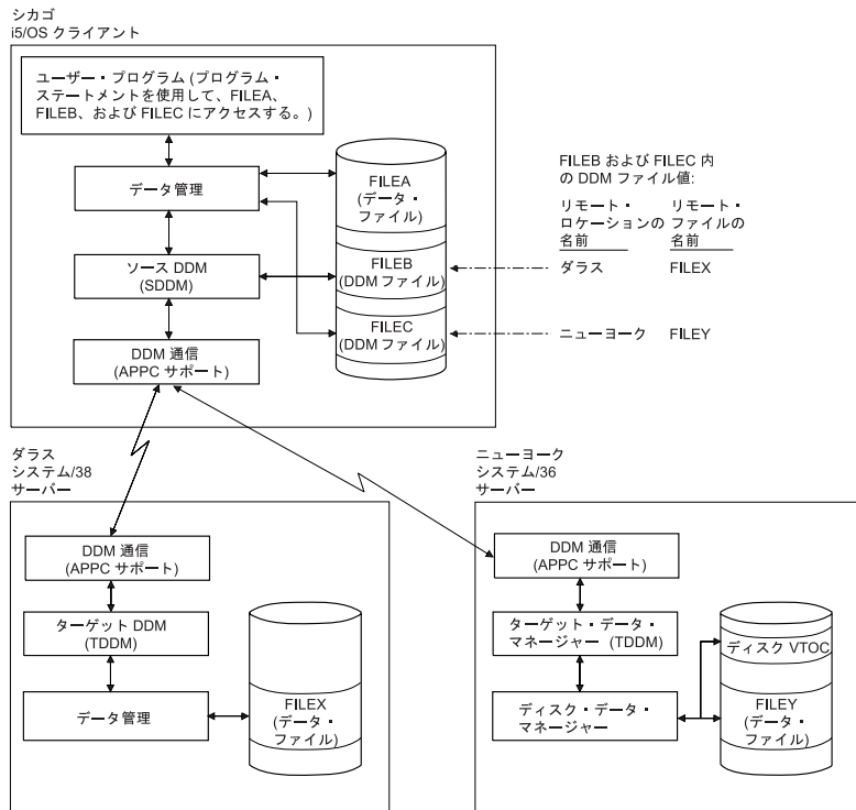
図 17. 例: 複数のローカルおよびリモート・ファイルへのアクセス: システム/38 およびシステム/36 との通信リンクを持った i5/OS。
