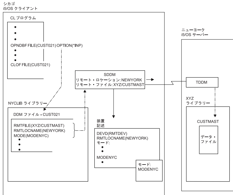
図 11. DDM ファイル・パラメーターとシステムとの関係
