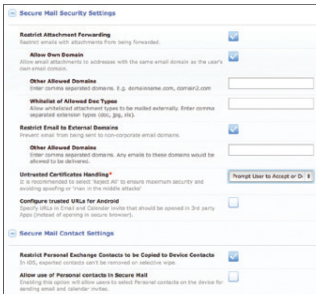
Рис. 2. Пример параметров безопасности для MaaS360 Secure Mobile Mail
