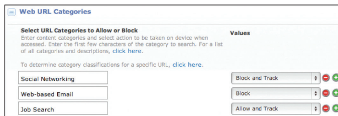
Figure 4 : Filtrage des catégories d'URL pour MaaS360 Secure Mobile Browser
