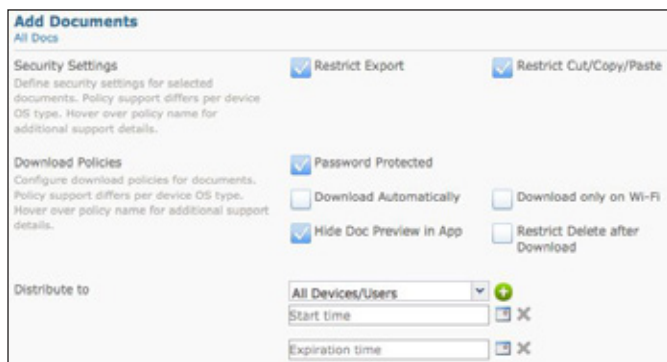
Figure 5 : Exemple d'options de création de règles en matière de gestion de document
