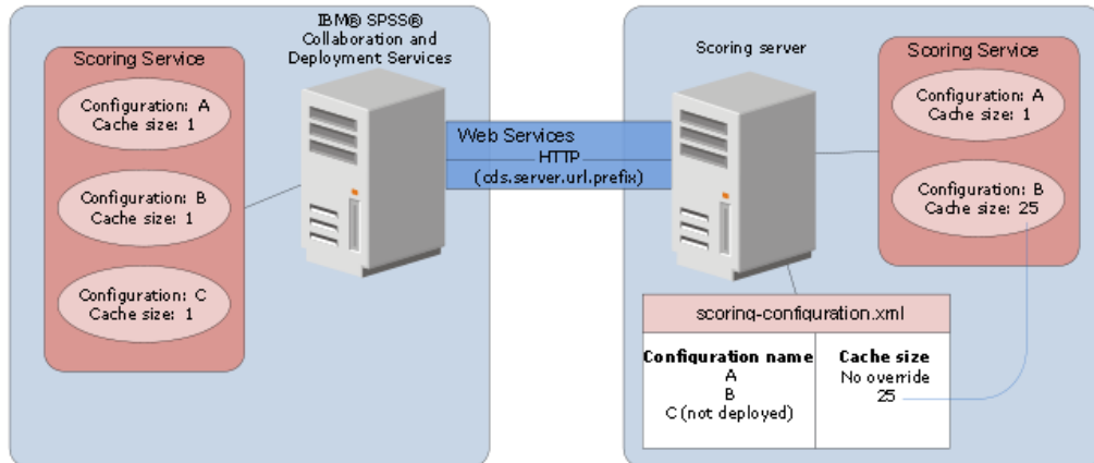
圖 4. 評分伺服器環境配置
