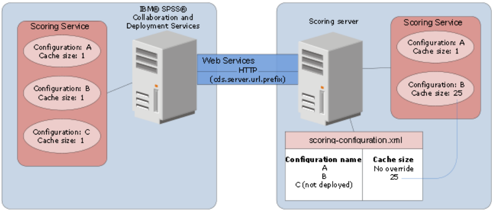
图 4: 评分服务器环境配置
