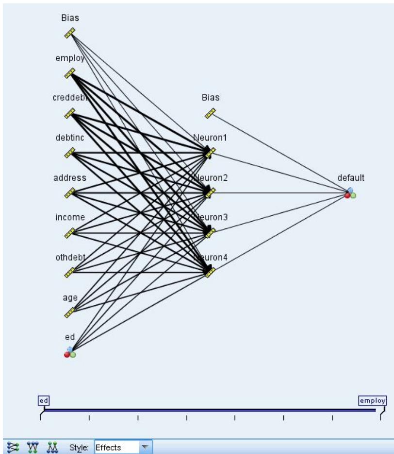
Рисунок 42. Представление сети, входные поля слева, стиль эффектов
