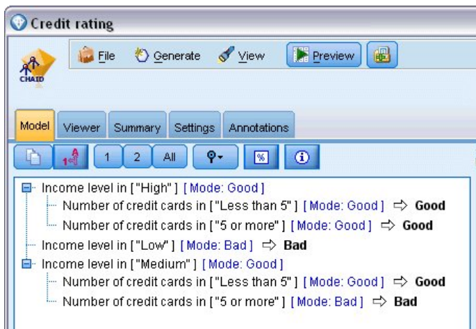
Рисунок 9. Слпок модели CHAID, набор правил
