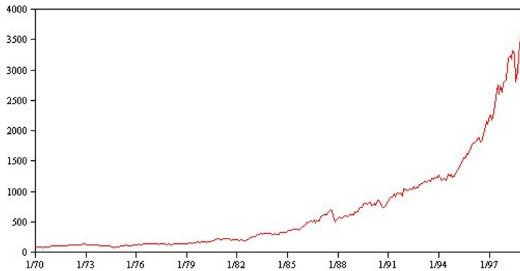
Рисунок 53. Тренд
