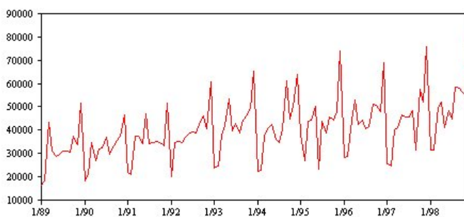
Рисунок 54. Сезонный цикл
