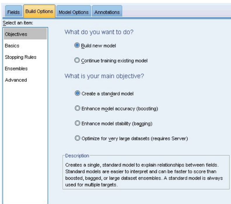
Рисунок 32. Целевые параметры
