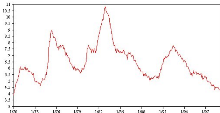
Рисунок 55. Несезонный цикл
