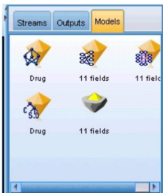
Рисунок 26. Палитра моделей
