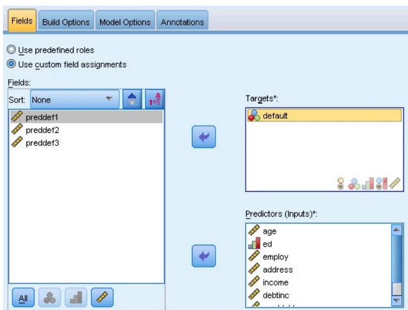
Рисунок 30. Вкладка Поля
