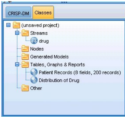
그림 9. 클래스 보기
