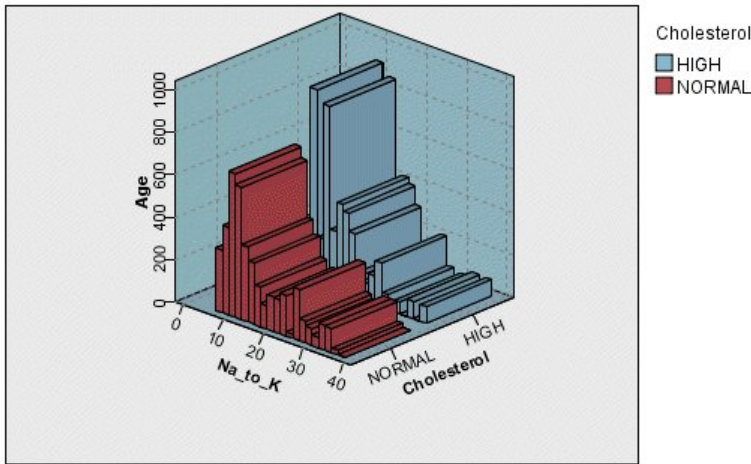
그림 33. 콜레스테롤 수준 높음 및 정상에 대해 연령에 대한 Na_to_K의 합계를 보여주는 3차원 컬렉션 그래프
