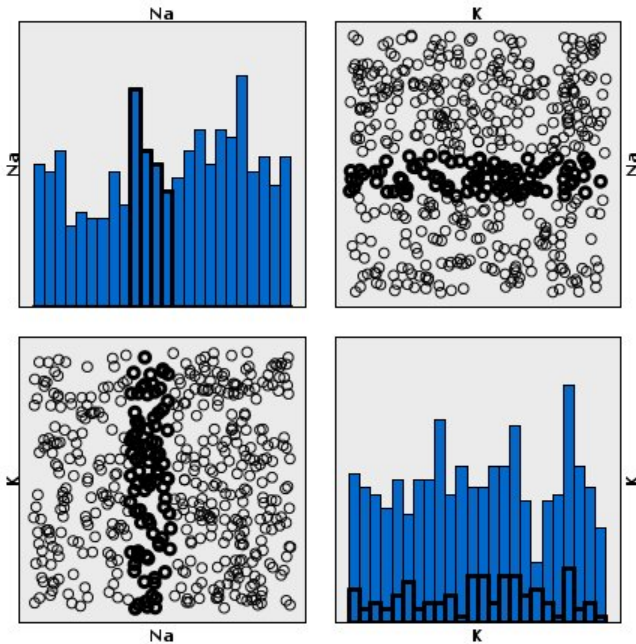
그림 69. SPLOM에서 요소 표시
