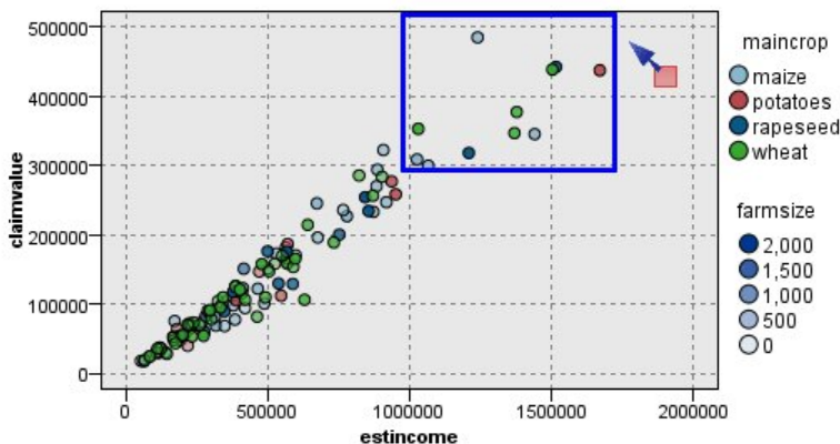
그림 65. 높은 클레임 값의 영역 정의
