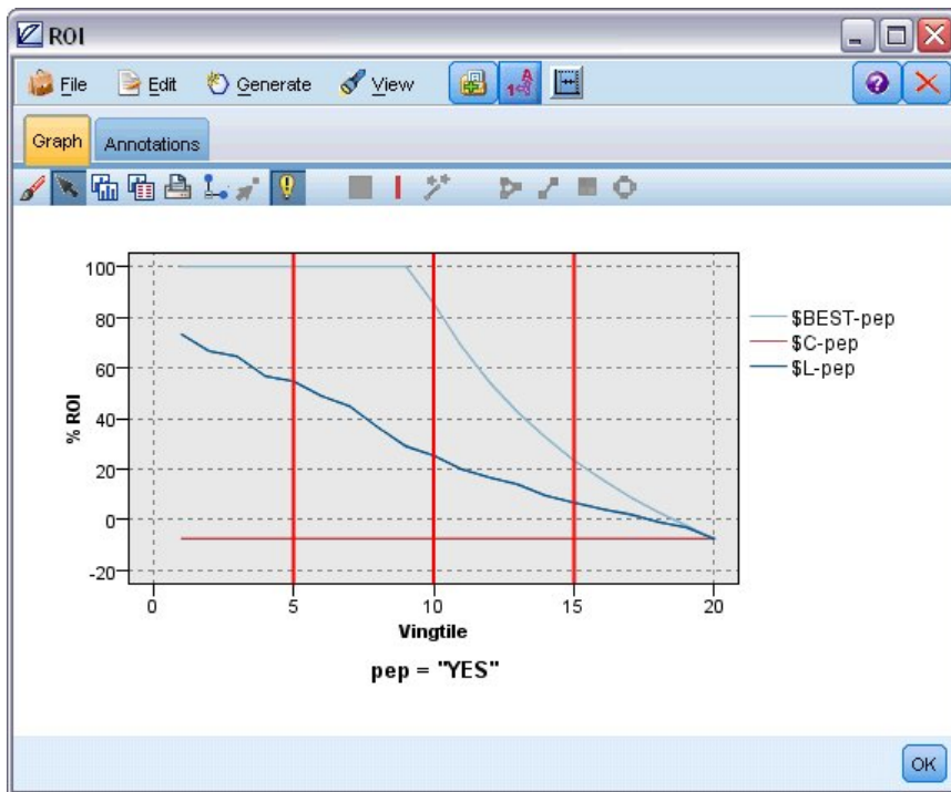
그림 59. 3개의 밴드가 있는 그래프
