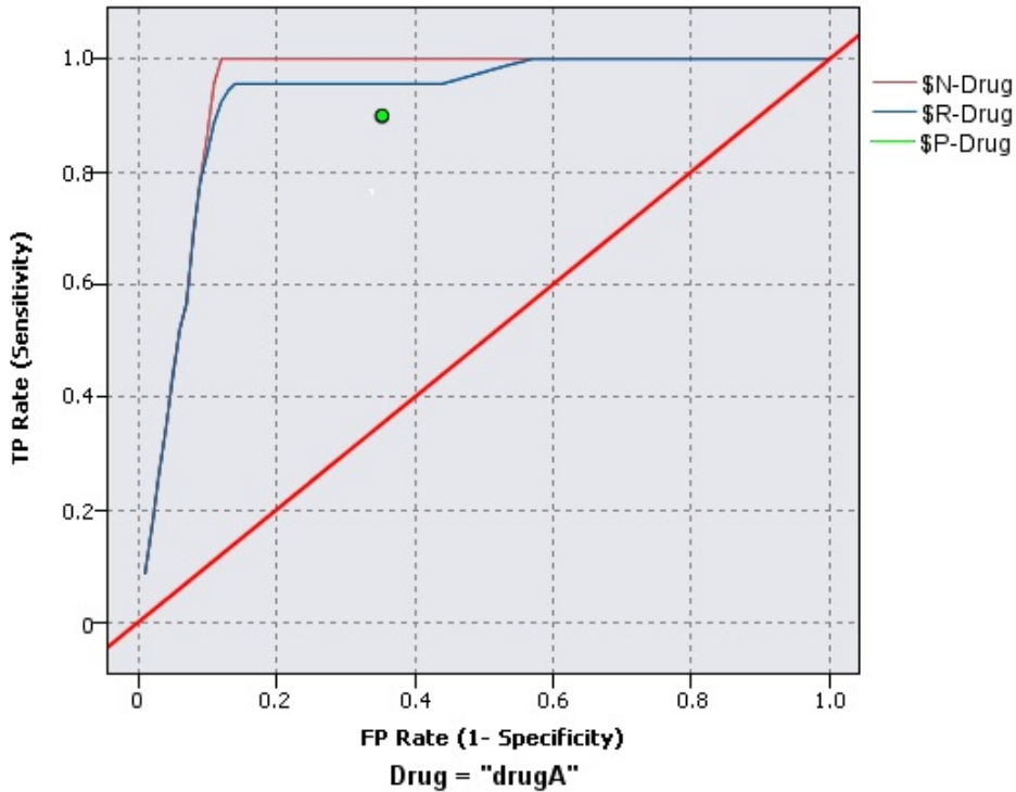
그림 46. 최적 예측선을 사용하는 ROC 차트
