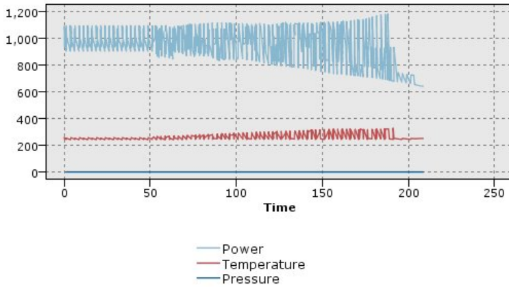
그림 24. 시간 경과에 따른 발전소 변동을 표시하는 표준 다중 도표(정규화를 수행하지 않으면 전압에 대한 도표를 볼 수 없음)
