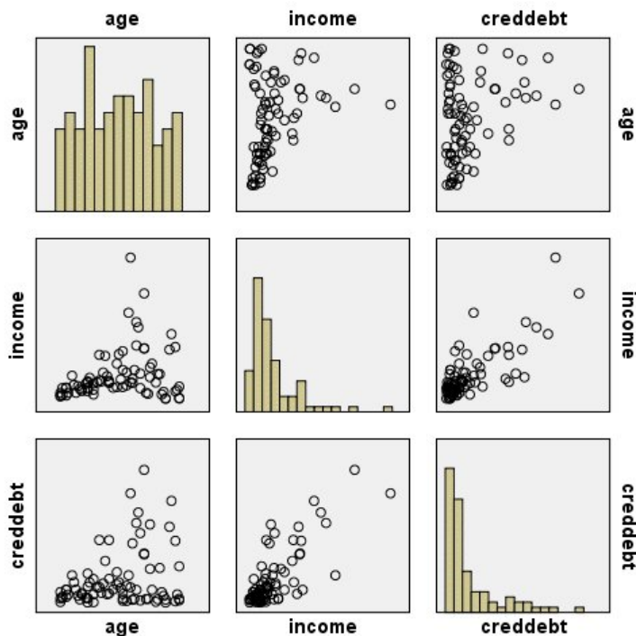
그림 15. 산점도 행렬(SPLOM)
