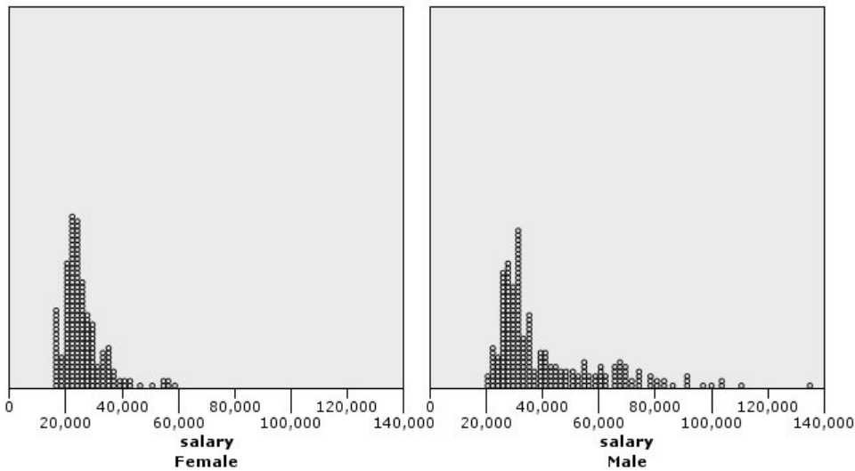
그림 11. 패넬링된 점도표
