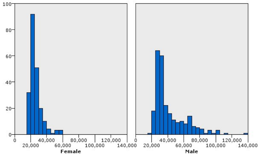
그림 10. 패널링된 히스토그램
