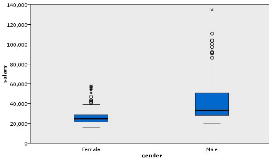
그림 12. 상자도표
