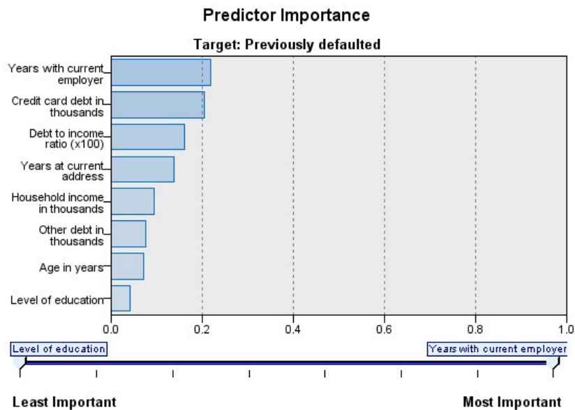
그림 39. 예측변수 중요도 보기
