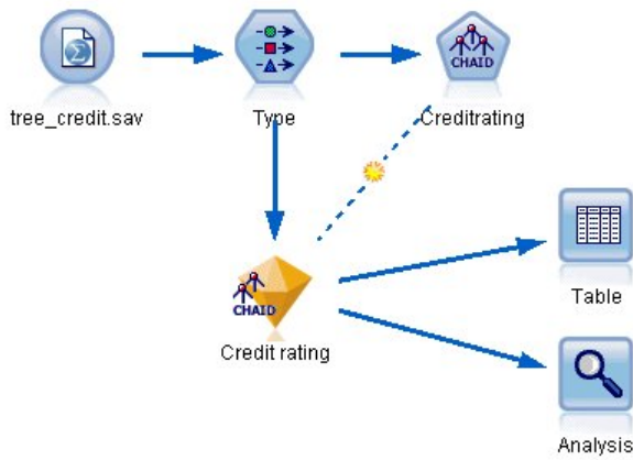
그림 14. 모델 평가를 위해 출력 노드에서 모델 너짓 첨부
