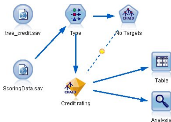
図 18. スコアリングのための新しいデータの追加
