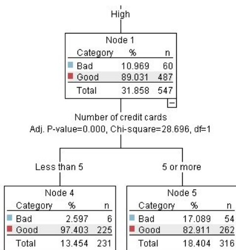
図 12. 高収入の顧客のツリー・ビュー
