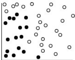
図 59. 元のデータセット
