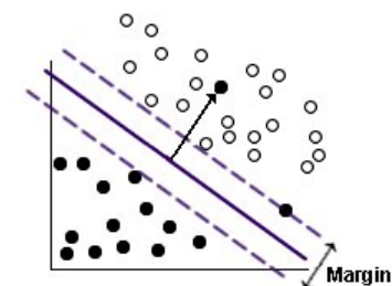
図 64. 線型区分の問題
