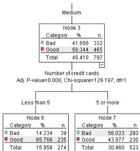
図 13. 中程度の収入の顧客のツリー・ビュー
