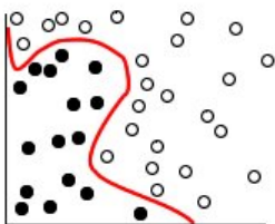
図 60. 区切りを追加したデータ
