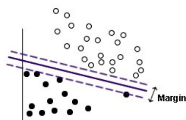
図 62. 予備的モデルを含むデータ
