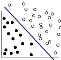
図 61. 変換されたデータ
