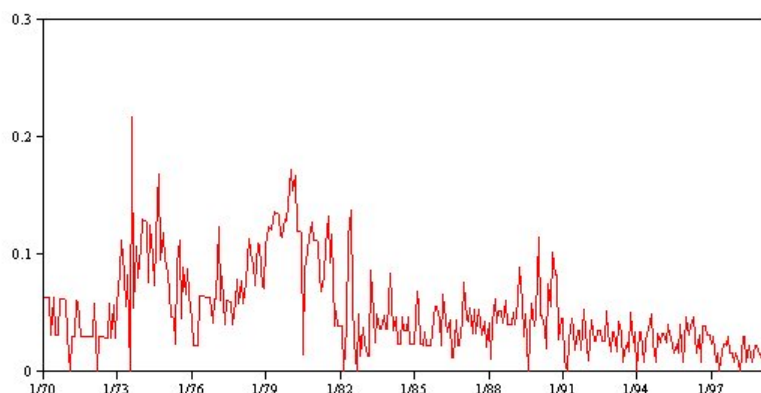
図 56. パルスが含まれる時系列
