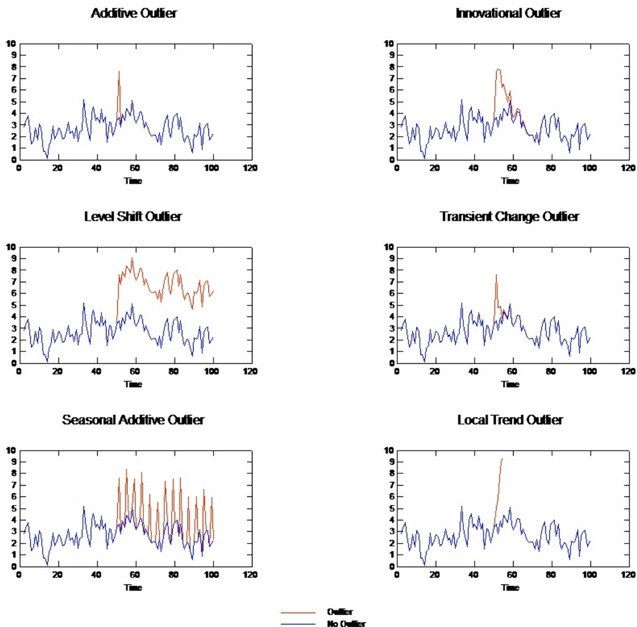
図 57. 外れ値のタイプ
