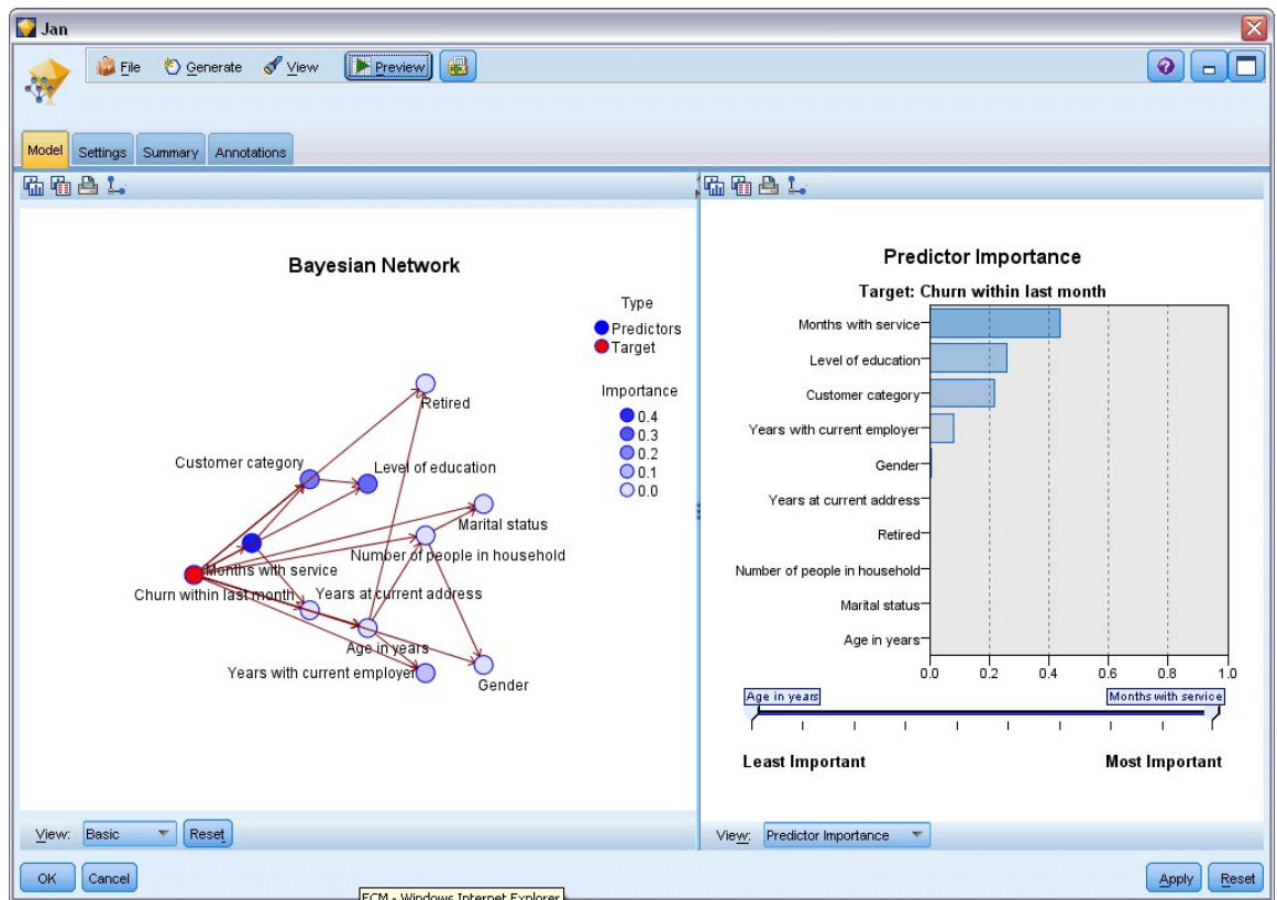
Figure 250. Modèle Réseau Bayésien montrant l'importance des prédicteurs
