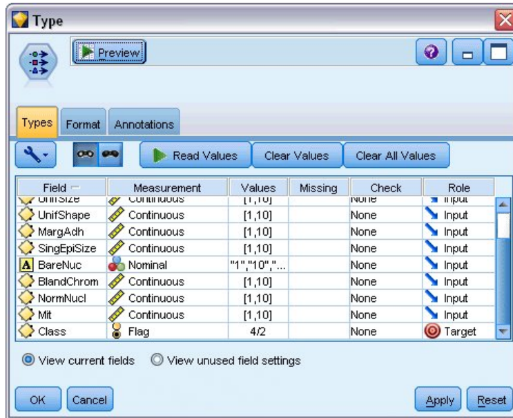
Figure 329. Paramètres du noeud type
