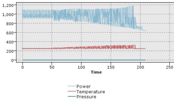
Figura 24. Gráfico múltiple estándar que muestra la fluctuación de la planta de energía durante un período de tiempo (tenga en cuenta que sin la normalización, resulta imposible ver el gráfico Pressure)
