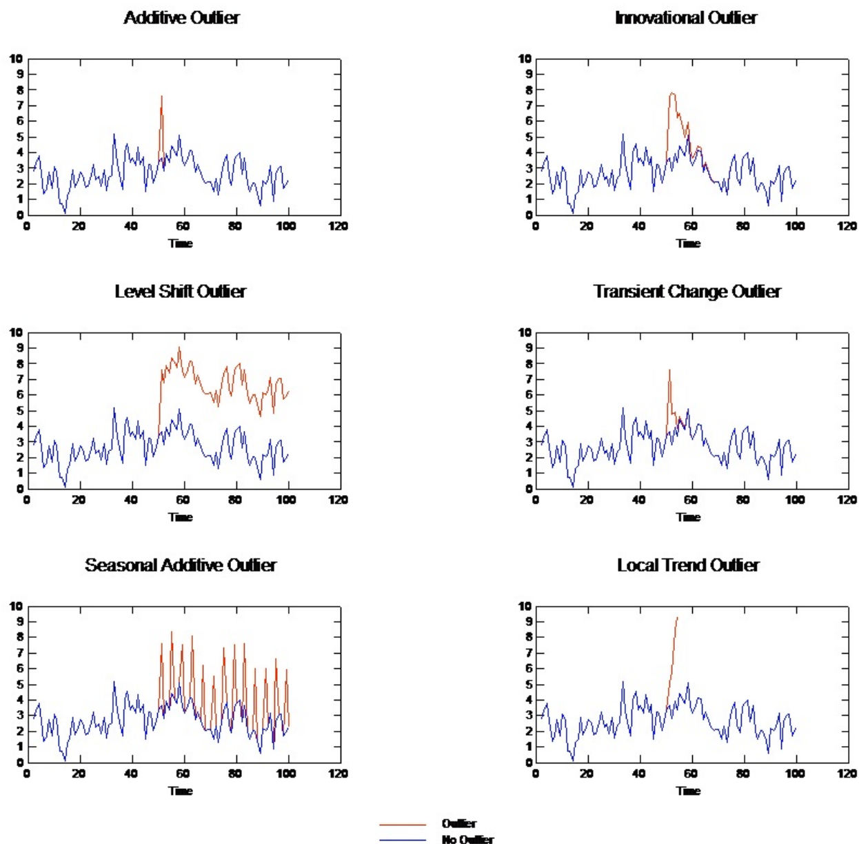
Figura 57. Tipos de valor atípico
