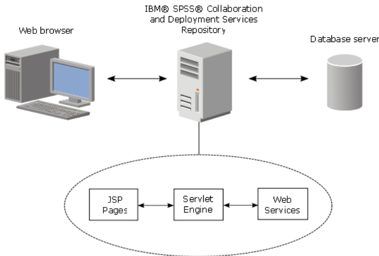
Abbildung 1. JSP-Architektur
