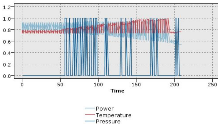
Abbildung 25. Normalisierter Multiplot mit einem Plot für den Druck (Pressure)
