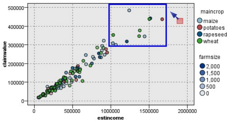
Abbildung 65. Definieren eines Bereichs mit hohen Forderungswerten
