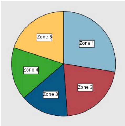
Abbildung 13. Kreisdiagramm
