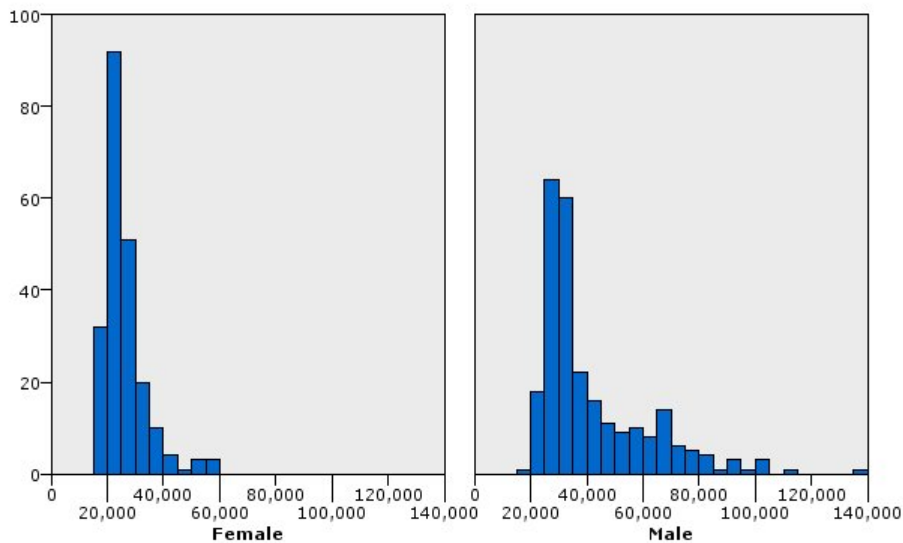
Abbildung 10. Unterteiltes Histogramm
