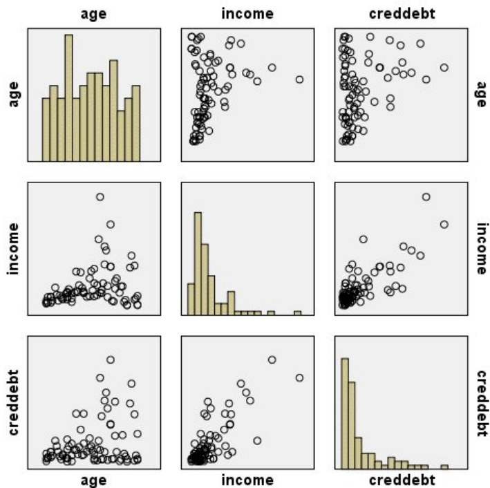
Abbildung 15. Streudiagrammmatrix (SPLOM)
