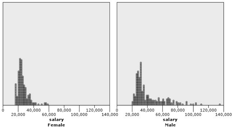
Abbildung 11. Unterteiltes Punktdiagramm
