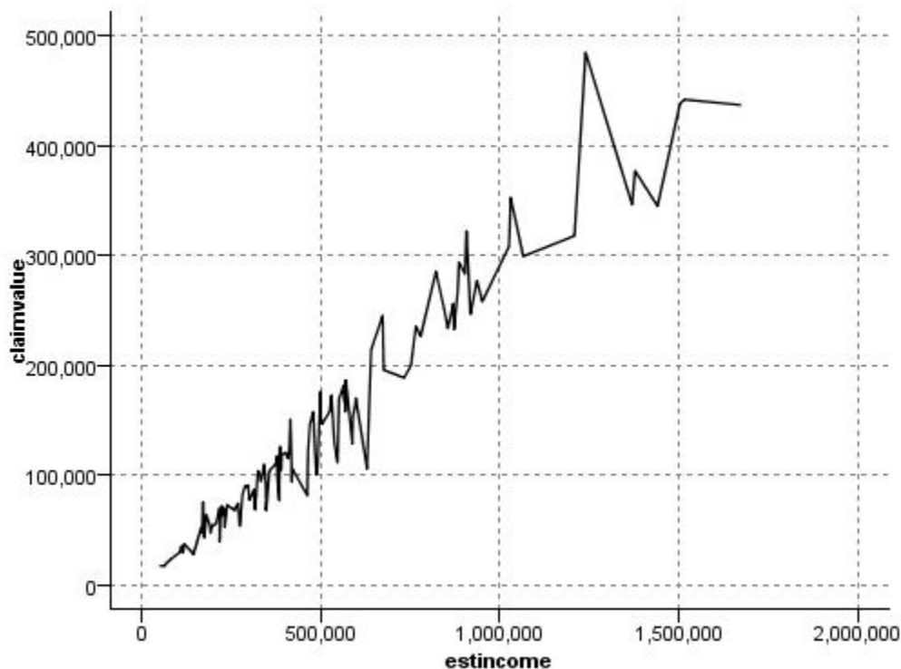
Abbildung 19. Liniendiagramm mit X-Modus "Sortieren"
