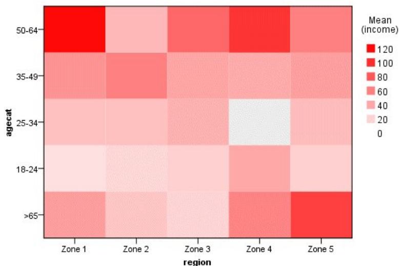
Abbildung 14. Kategoriale Heat-Map
