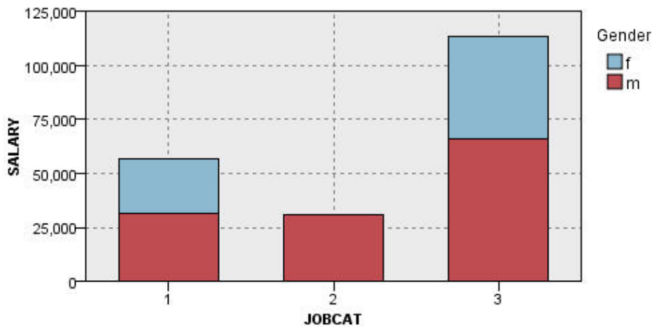
Abbildung 9. Gestapeltes Balkendiagramm
