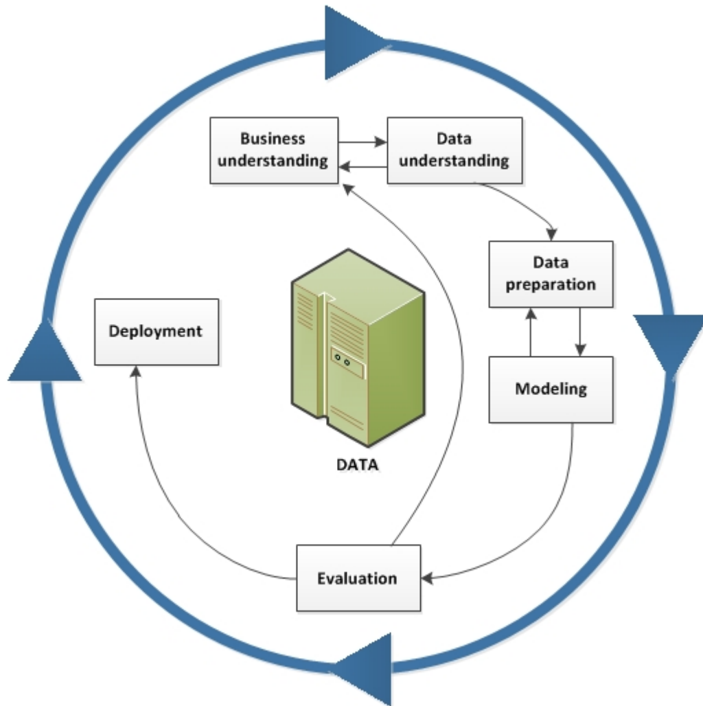
Abbildung 1. Data-Mining-Lebenszyklus
