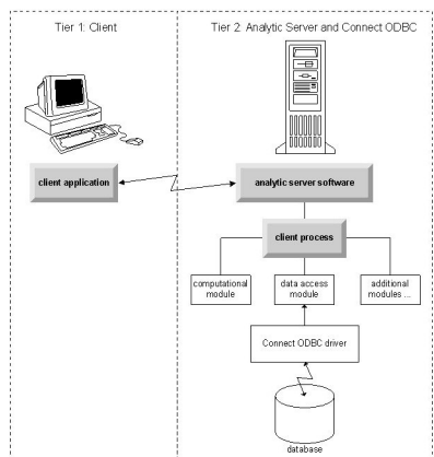
図 3. 分散分析モードでの Connect ODBC
