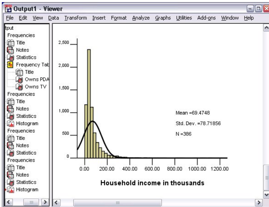
Figura 31. Histograma
