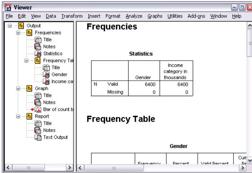
Figura 56. Visor
