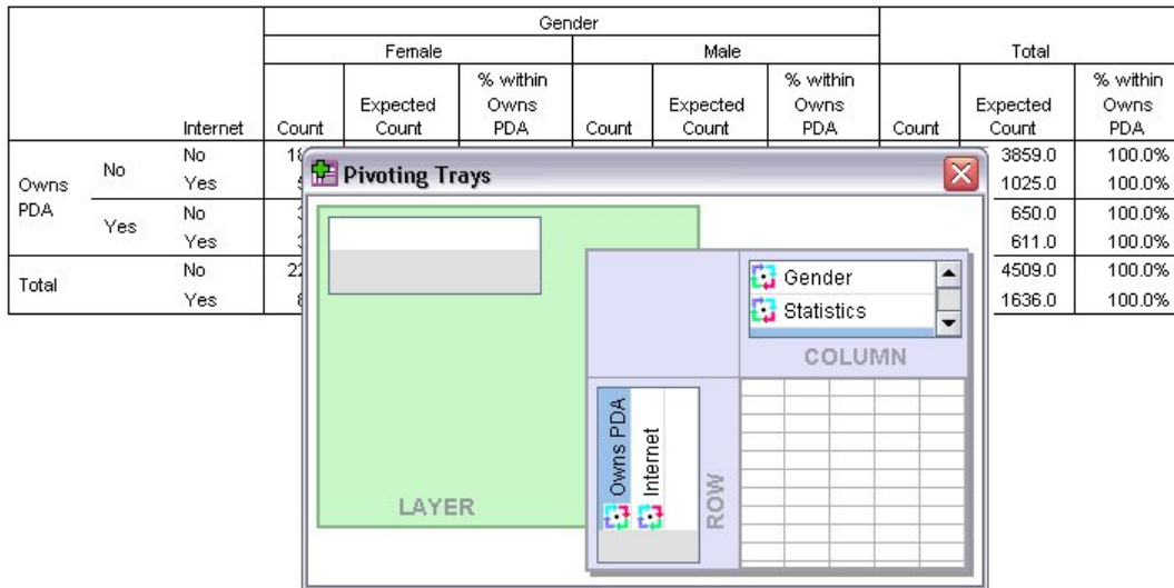
Figura 41. Intercambiar filas
