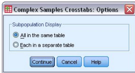
Abbildung 8. Dialogfeld "Optionen"
