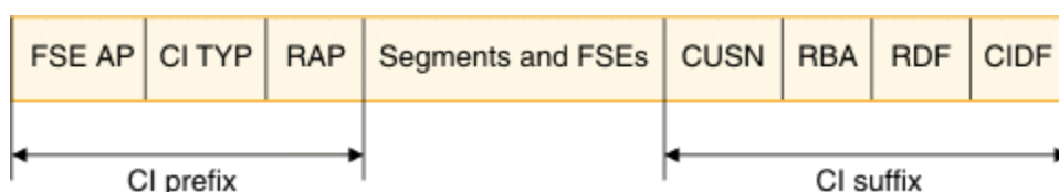
Figure 60. CI format
