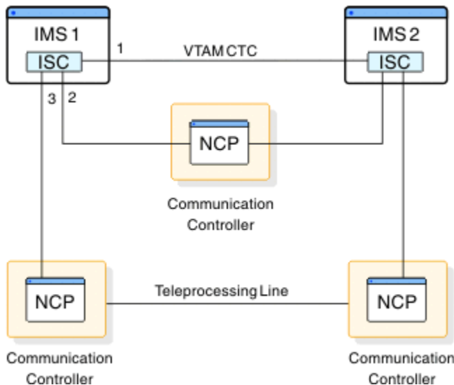
Figure 84. ISC link options
