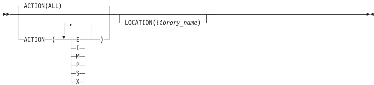
Figure 173. EDGSPLCS EXEC parameters
