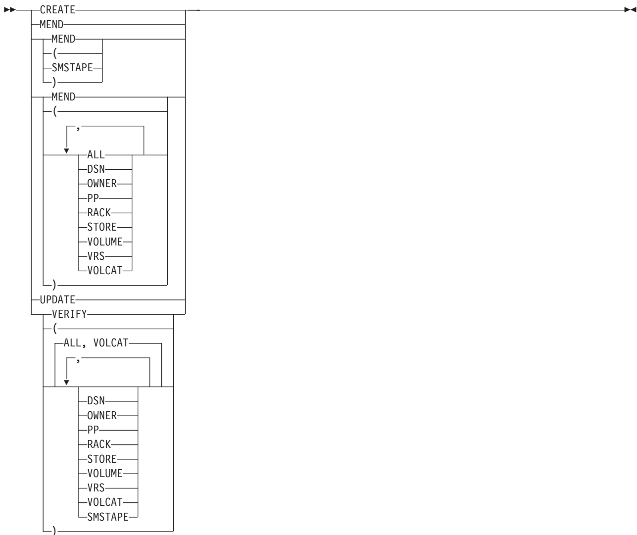
Figure 165. EDGUTIL EXEC parameters
